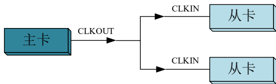
图 4-10-3 主从卡时钟级联同步采集的级联方式
