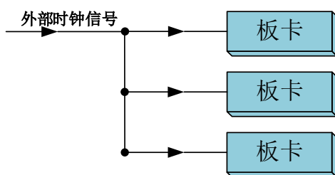
图4-10-5 外时钟同步采集的连接方式
