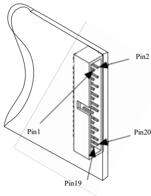
图 3-3-4 RTSI 的 Pinout 图
