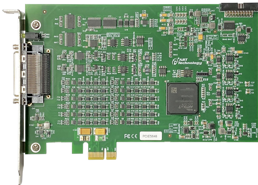
图 3-1-1 PCIe5648 板卡正面图
