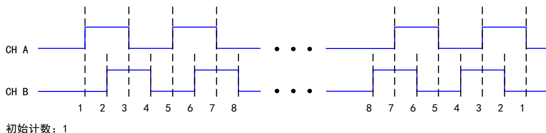
图 6-7-3 X4 编码
