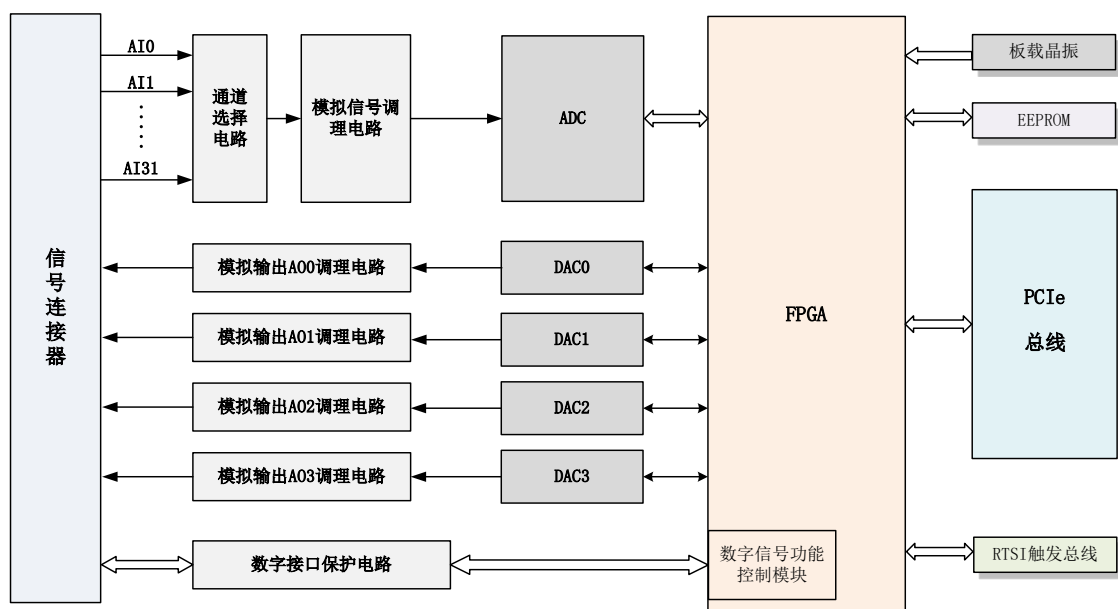
图2-2-1 PCIe5648系统框图
