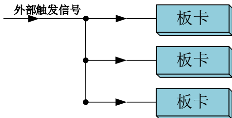
图 4-10-4 外触发同步采集的连接方式
