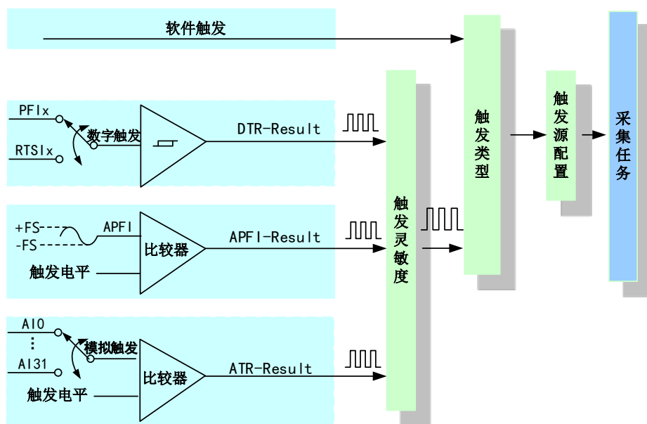
图 8-1-1 触发源选择
