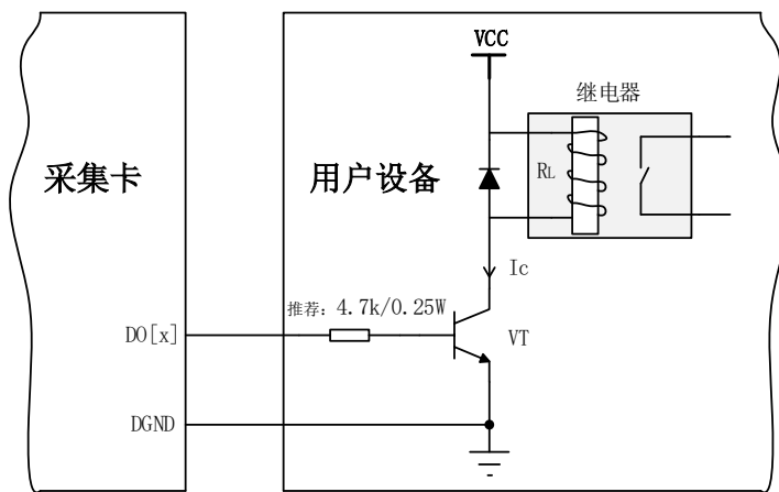
图 7-3-3 DO 数字量控制继电器电路
