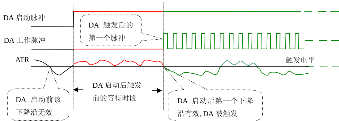
图 6.7 下降沿触发图例，上升沿同理
