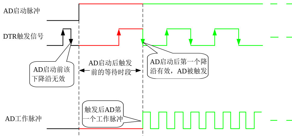
5.4 下降沿触发图例
