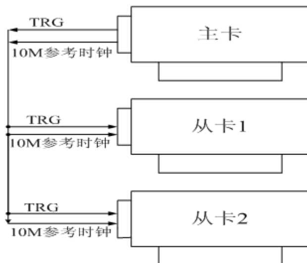
多卡级联的连接方法
